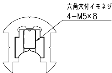
使用時の納まり S=1/1
