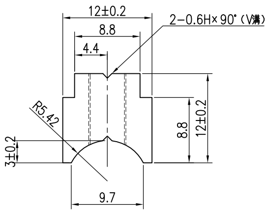
断面図 S=2/1
