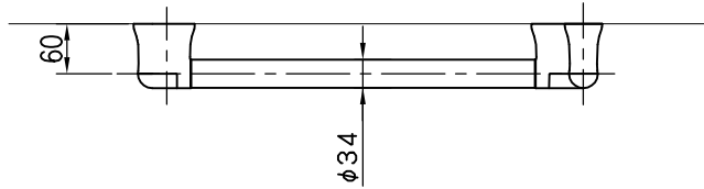
取付座詳細図 S=1/2
