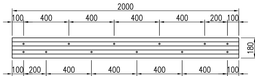
アンカーボルトピッチ (mm) S = 1/20
