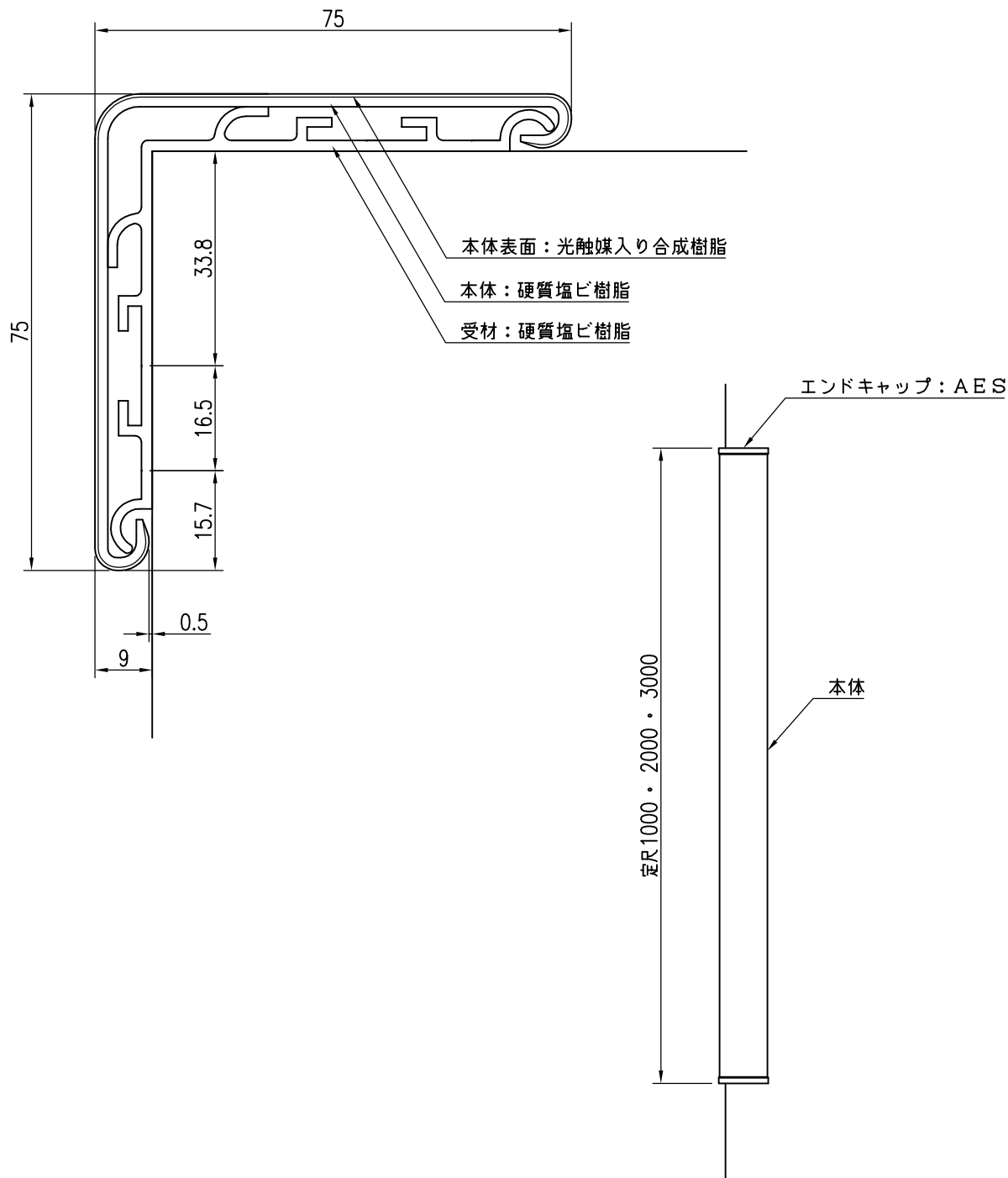
立面図 S=1/10
