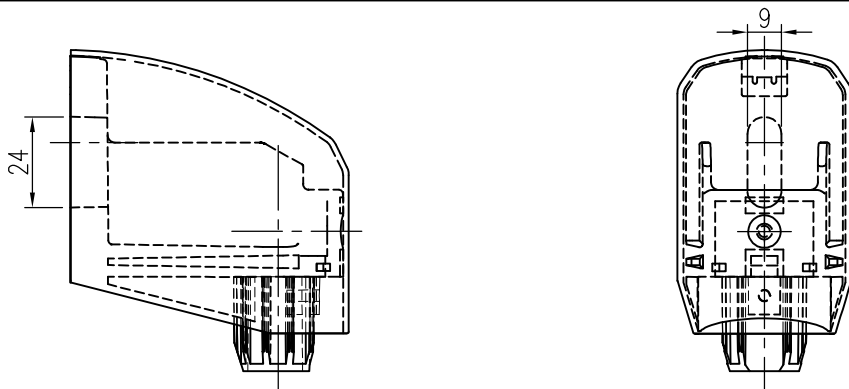
取付座詳細図 S=1/2
