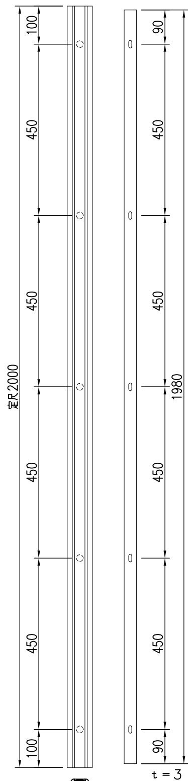
本体及び固定金具穴ピッチ S = 1 / 10
