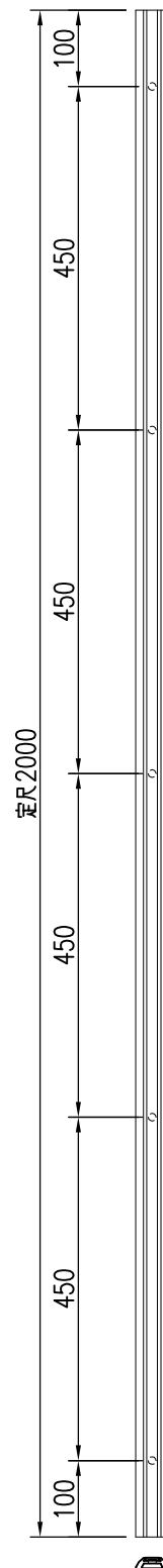
本体及び固定金具穴ピッチ S = 1 / 10
