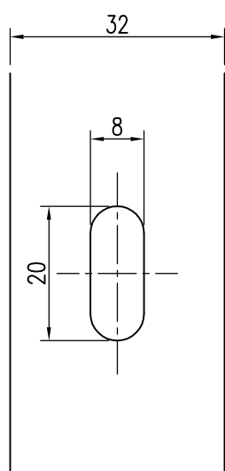
固定金具穴寸法 S = 1 / 1
