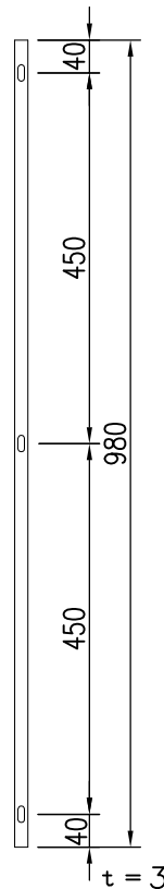
本体及び固定金具穴ピッチ S = 1 / 10
