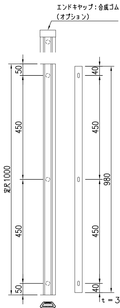
本体及び固定金具穴ピッチ S = 1 / 10
