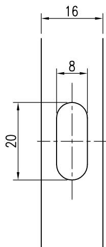
固定金具穴寸法 S = 1 / 1
