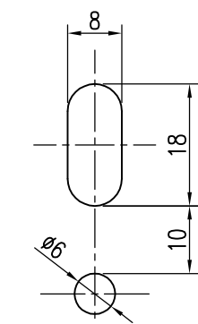
穴寸法 S = 1 / 1
