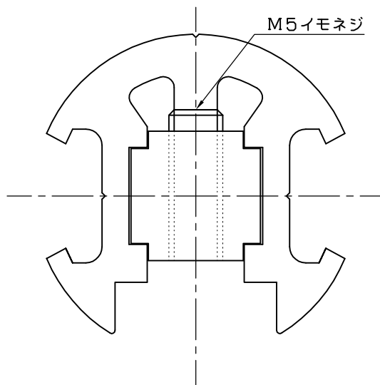
納まり図
