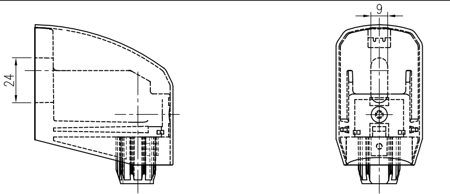
取付座詳細図 S=1/2
