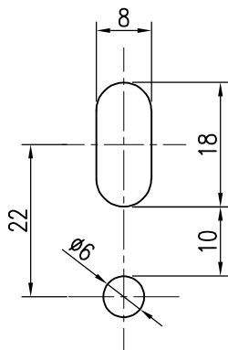
穴寸法 S = 1 / 1
