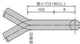
立寸法詳細図
