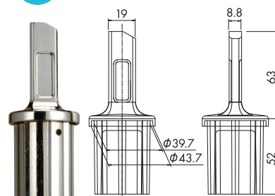
φ42.7 φ42.7用(パイプ肉厚1.5mm)
