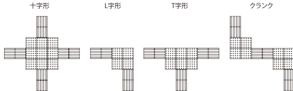
比較的広い場所での配置例（□300：線状鉋4本 / 点状鉋25個）
