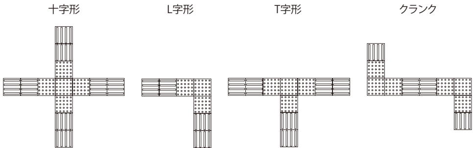
通常の配置例（□300：線状鉋4本 / 点状鉋25個）
