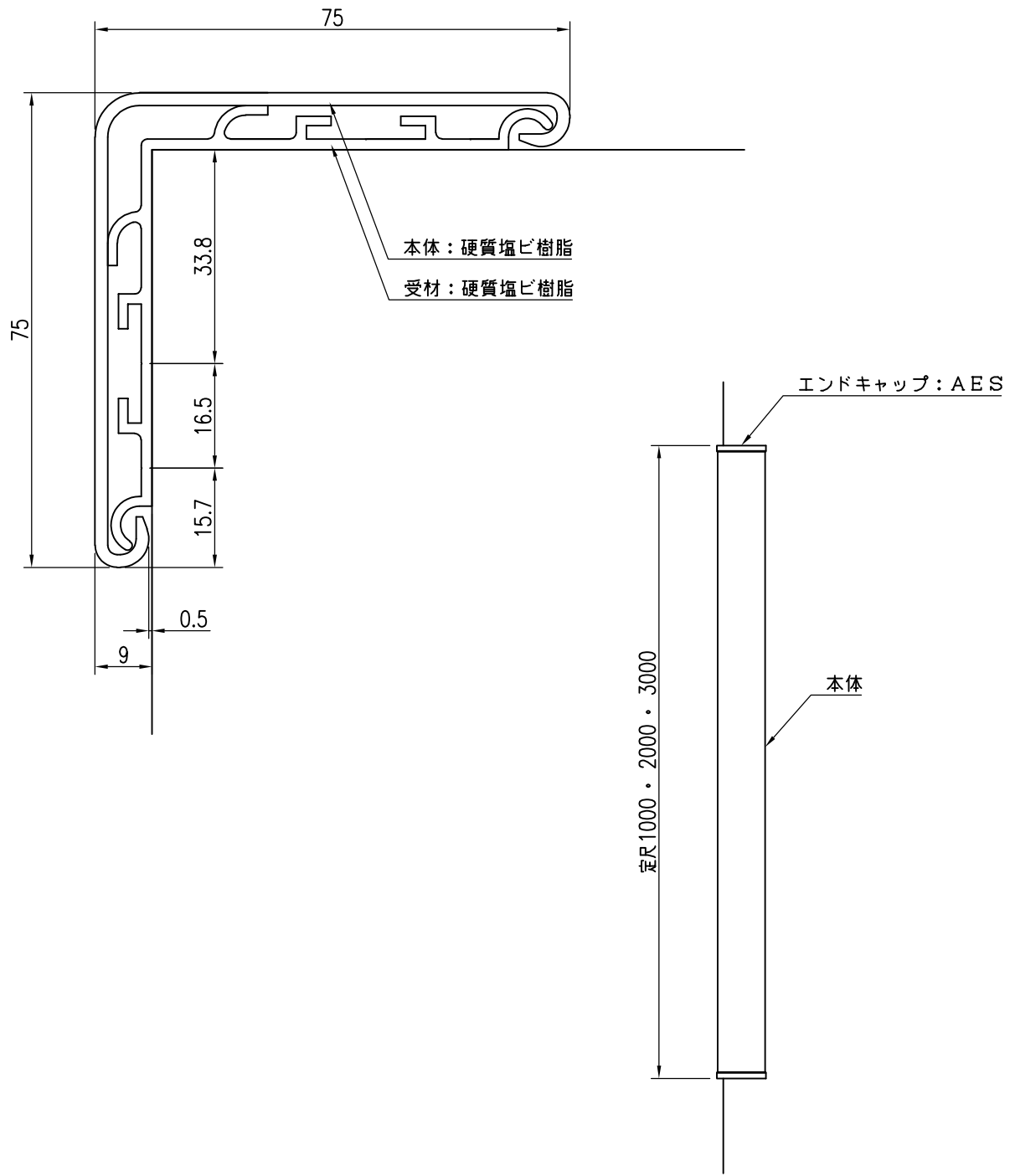
立面図 S=1/10
