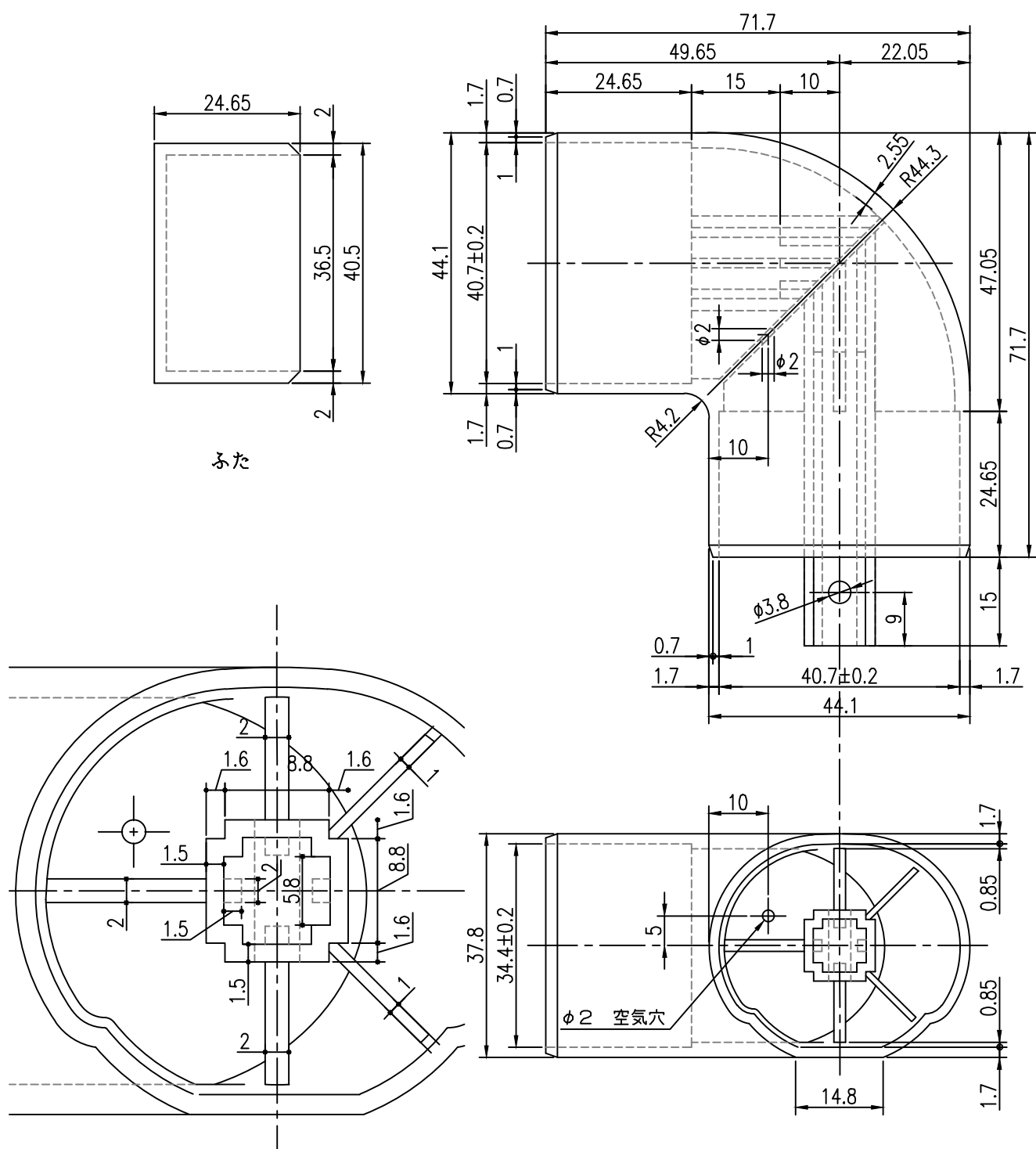
部分詳細図 S=2/1
