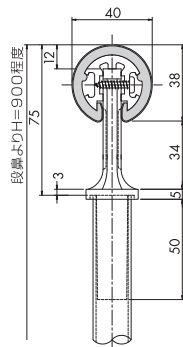
φ19・φ22用納り図
