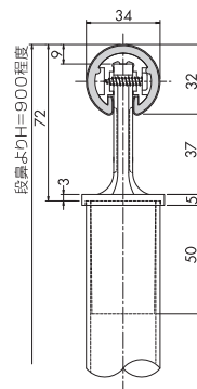
φ34・φ38・φ42.7用納り図
