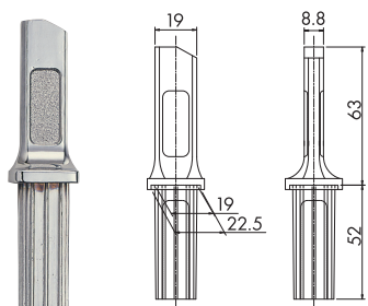
角22 □22用 (パイプ肉厚1.5mm)
