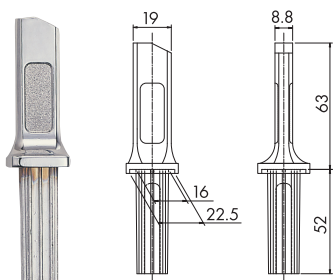
角19 □19用 (パイプ肉厚1.5mm)
