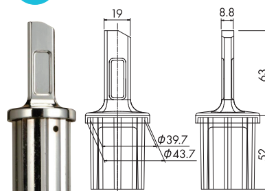
φ42.7 φ42.7用 (パイプ肉厚1.5mm)
