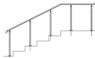
《アプローチ階段手すり設置例》
