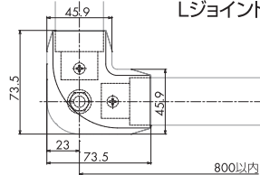
Lジョイントブラケット
