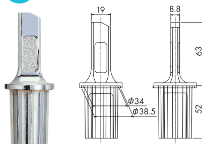
φ38 φ38用 (パイプ肉厚2.0mm)
