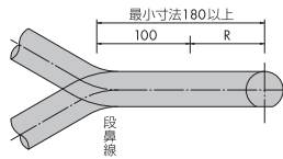
立面寸法詳細図
