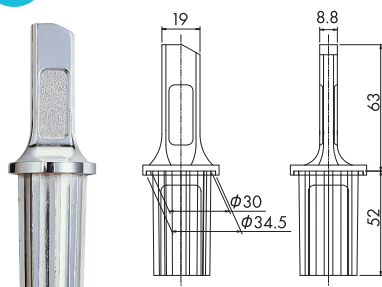
φ34 φ34用 (パイプ肉厚2.0mm)
