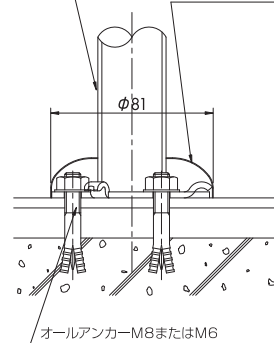
φ42.7 φ42.7用 (パイプ肉厚1.5mm)
