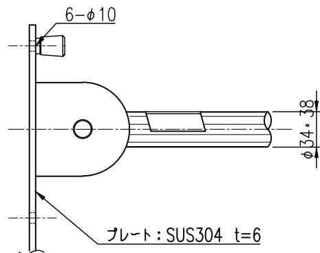
取付座詳細図 S=1/5
