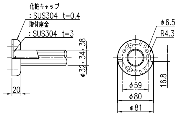
取付座詳細図 S=1/5
